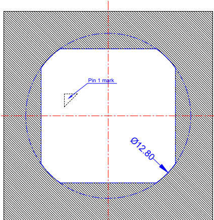
Top View 阴影部分为可切割区域
